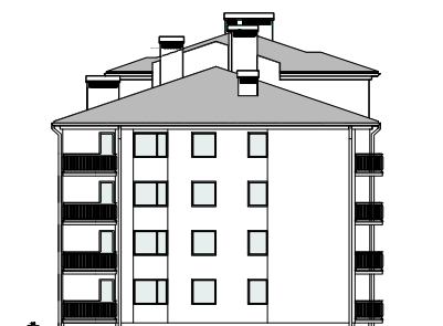
ELEWACJA ZACHODNIA
